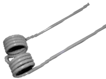
• 270050120 Пресс-подборщик KRONE Диаметр проволоки: 5,5 мм
