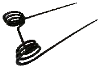
• 143113/143112 Тяжелая борона DEGELMAN Диаметр проволоки: 16,0 мм/14,0 мм
