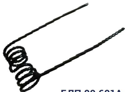
• БЛП.00.601А Средняя борона ЮГЖЕЛДОРМАШ Диаметр проволоки: 10,0 мм
